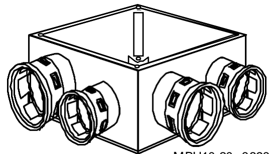
MBH10-20, 089019
